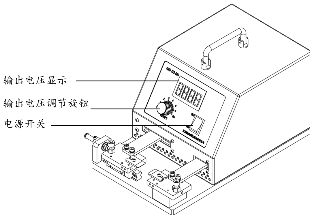
E 型-500W 便携式阻抗焊机 控制显示面板
