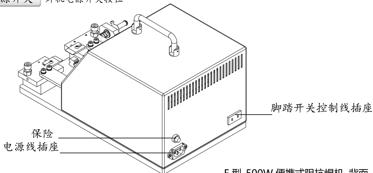
E 型-500W 便携式阻抗焊机 背面
