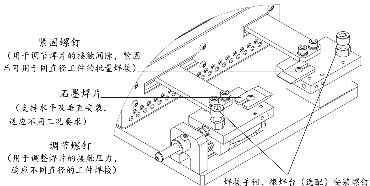
焊接平台功能简介
