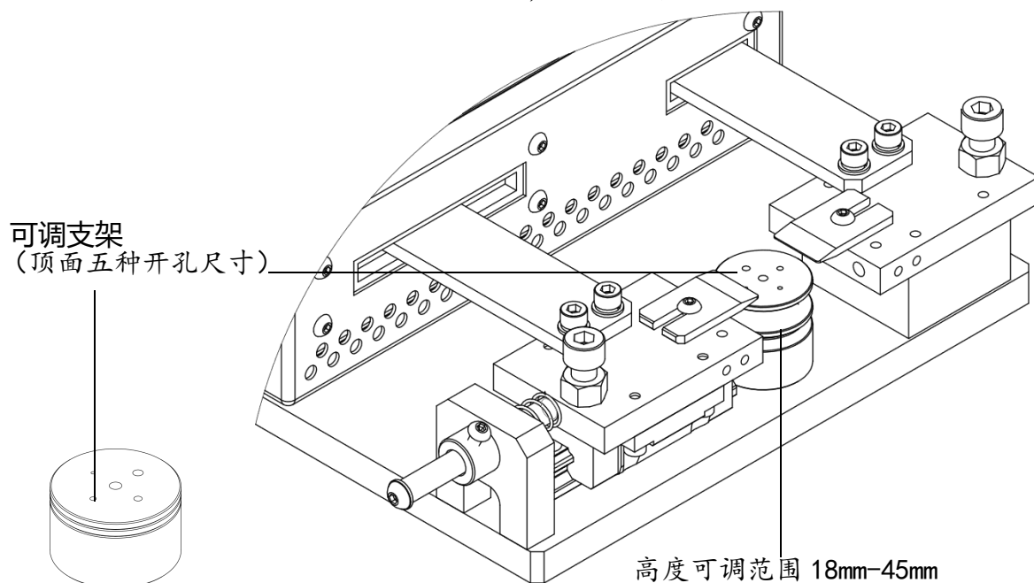
可选工装-可调支架在 E 型焊机上的使用示意
