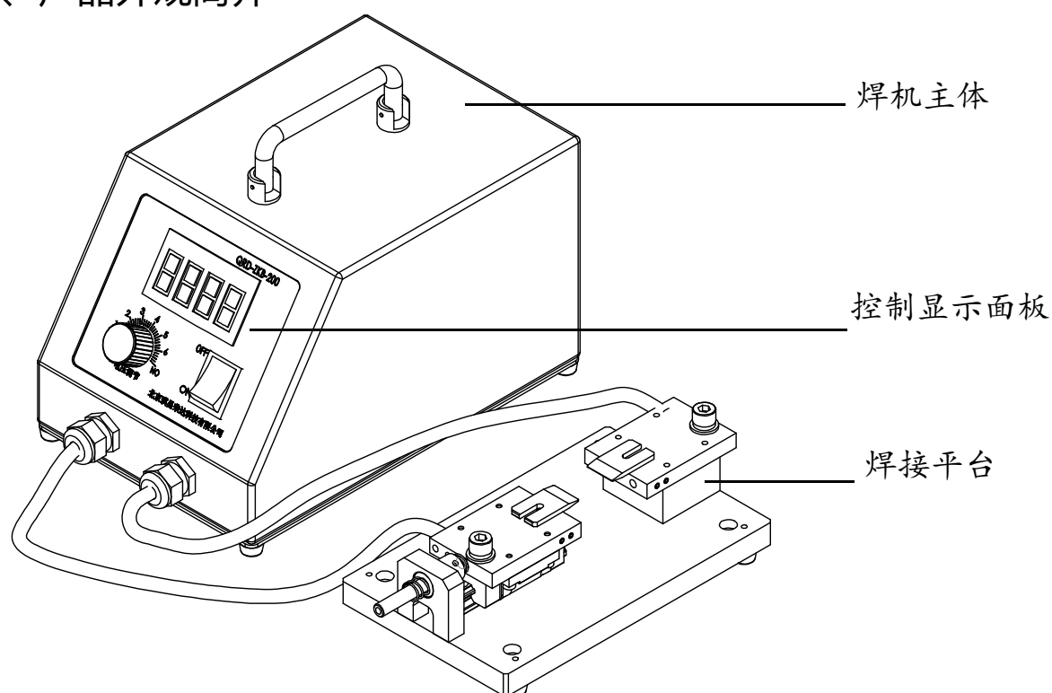
B 型-200W 便携式阻抗焊机 总图
