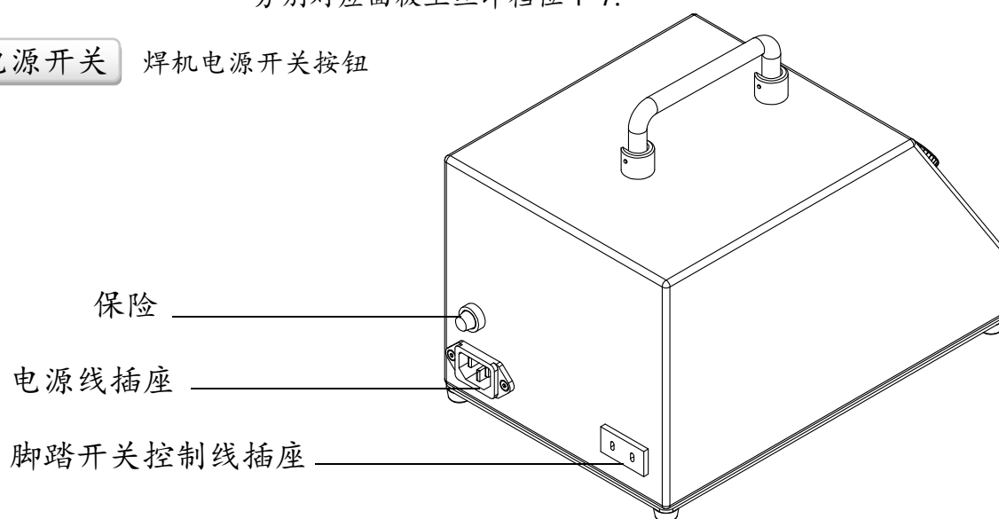
B 型-200W 便携式阻抗焊机 背面
