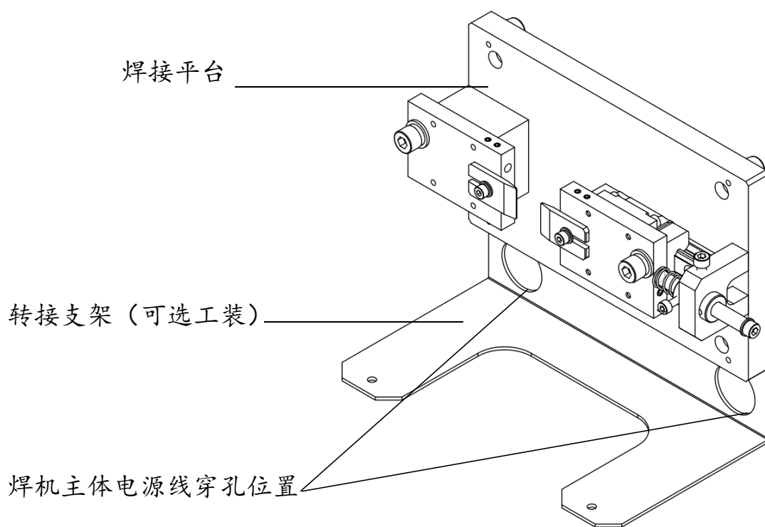
焊接平台竖向安装示意
