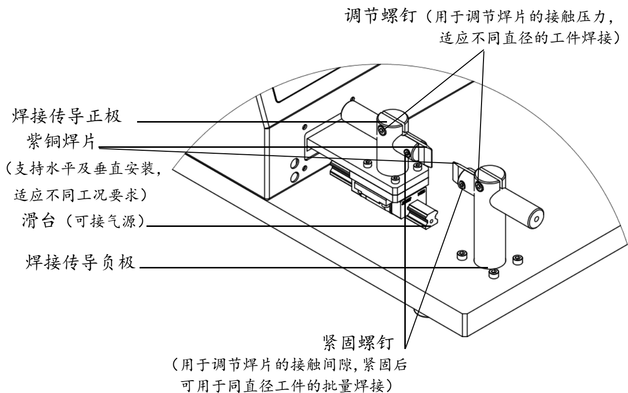
A 型-2000W 台式阻抗焊机 焊接传导装卡装置部分
