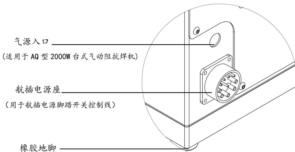
A 型-2000W 台式阻抗焊机 背面
