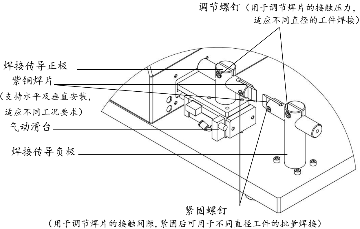
AQ 型-2000W 台式阻抗焊机 焊接传导装卡装置部分
