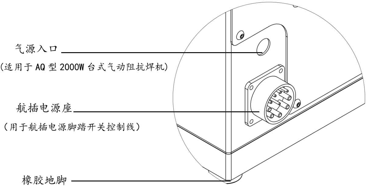
AQ 型-2000W 台式阻抗焊机 背面
