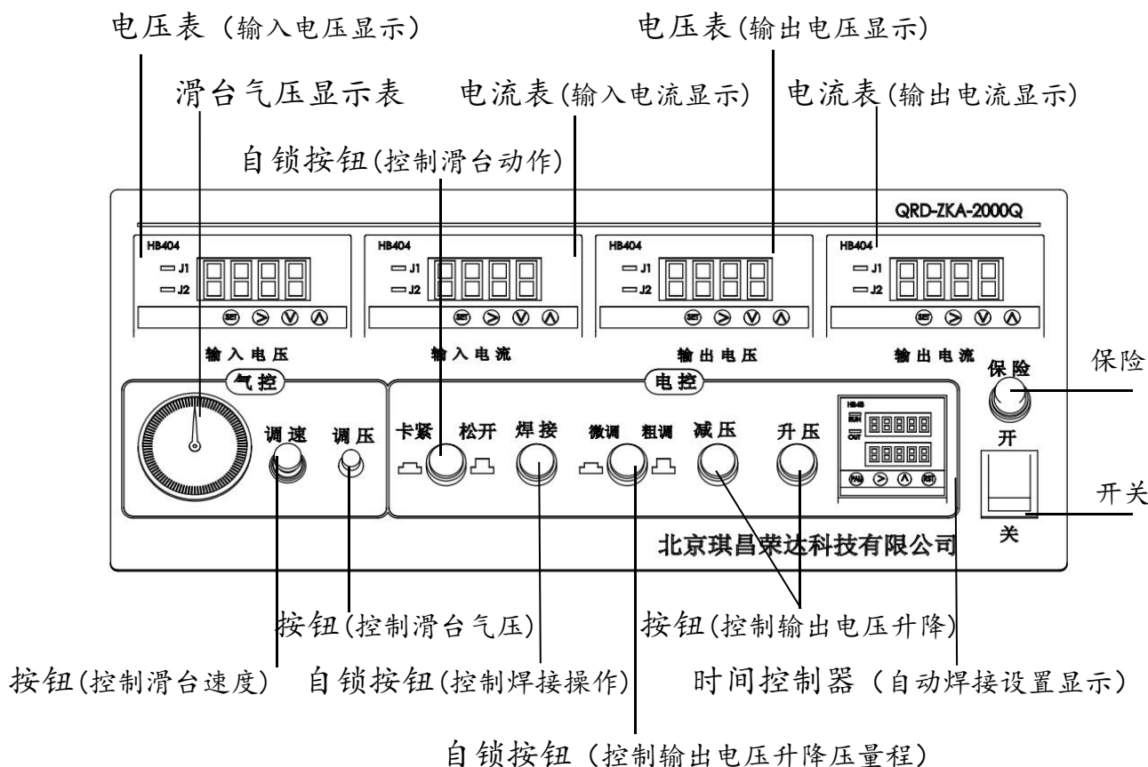
AQ 型-2000W 台式阻抗焊机 控制显示面板
