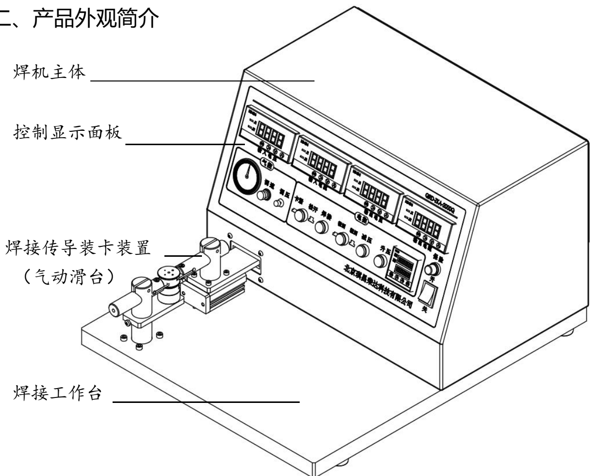
AQ 型-2000W 台式阻抗焊机 总图
