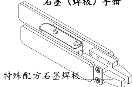
石墨（焊极）手钳
